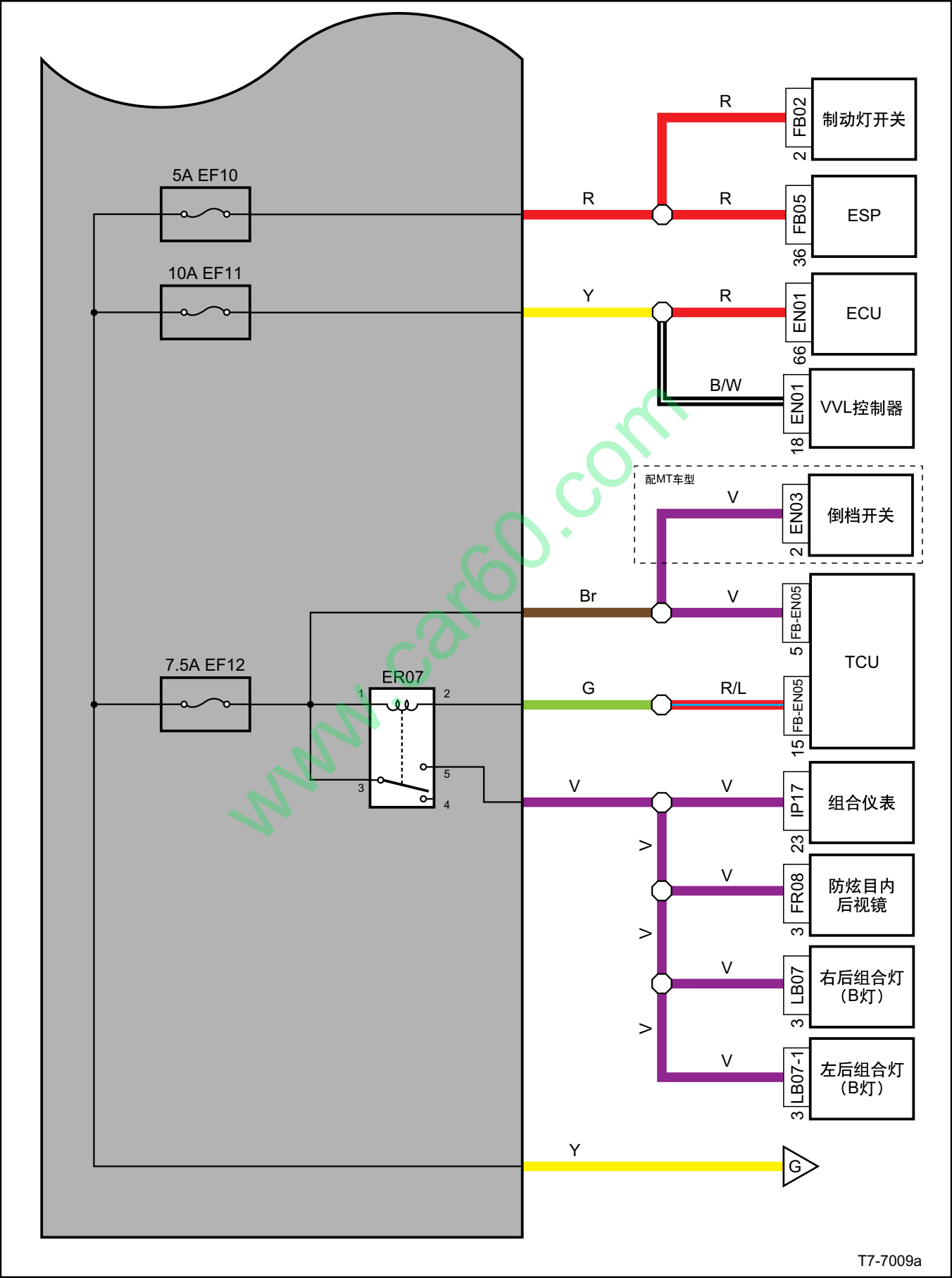
前机舱保险丝、继电器电源分布图（续8）
