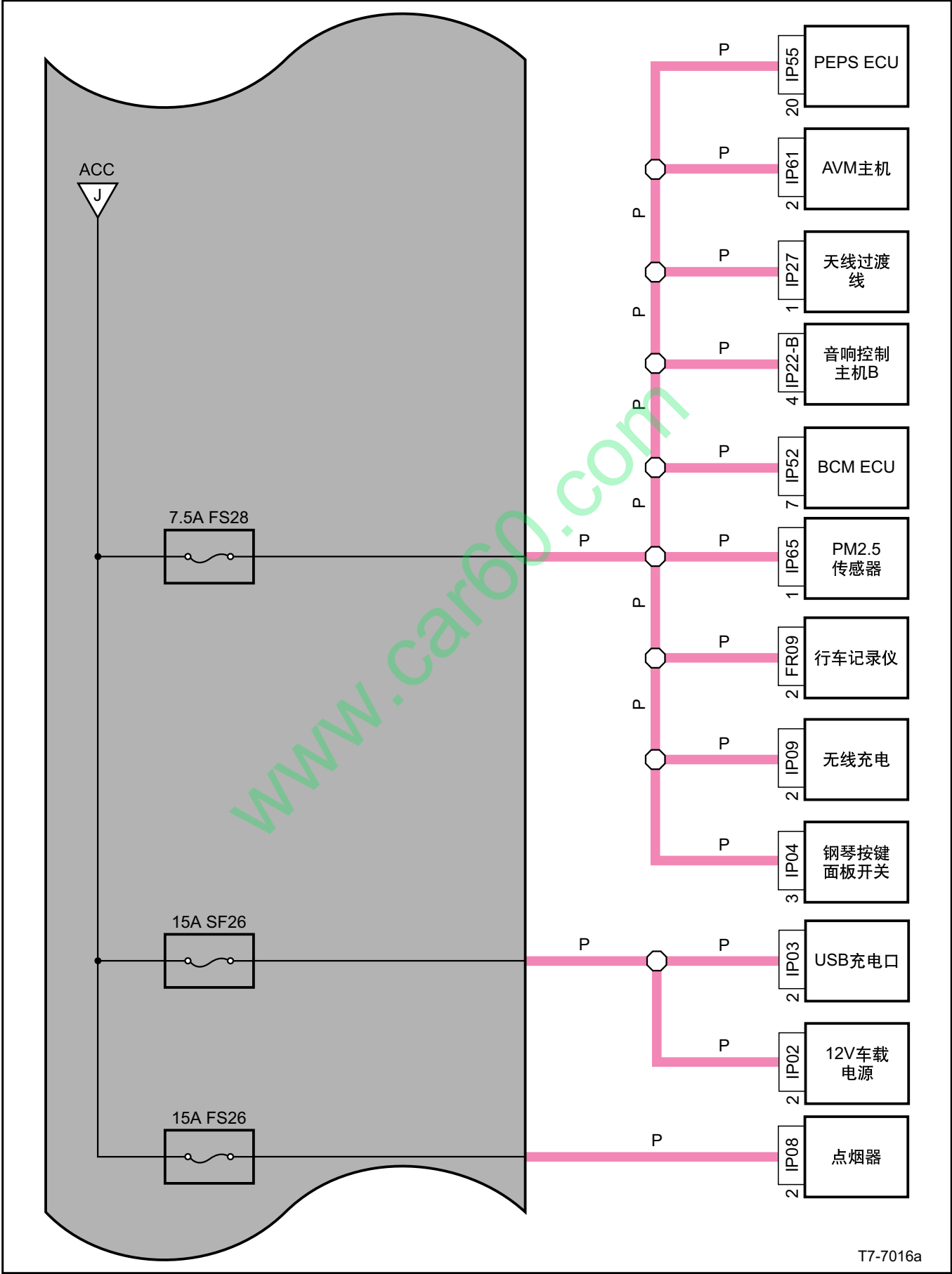
室内保险丝、继电器电源分布图（续6）
