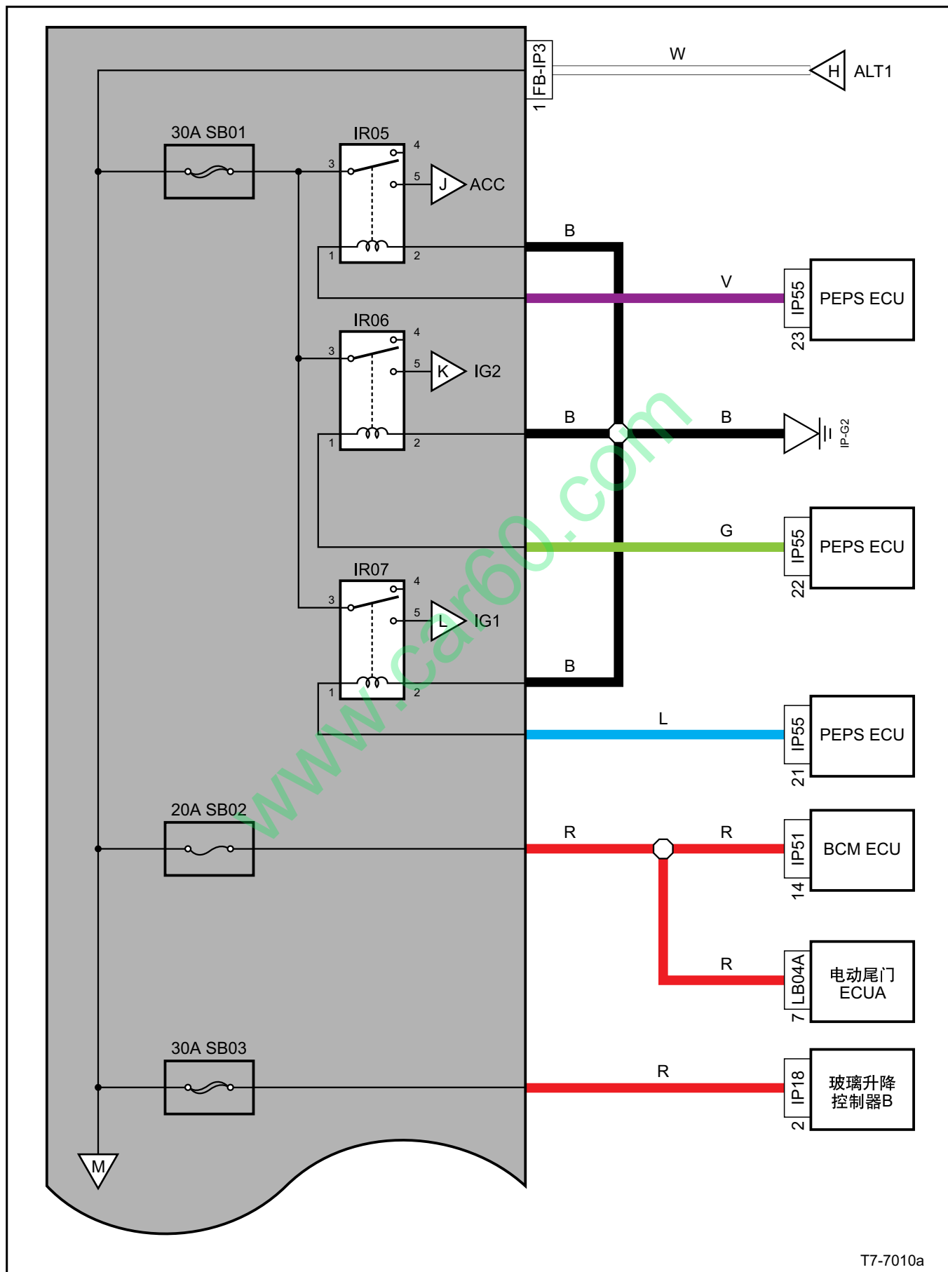
室内保险丝、继电器电源分布图
