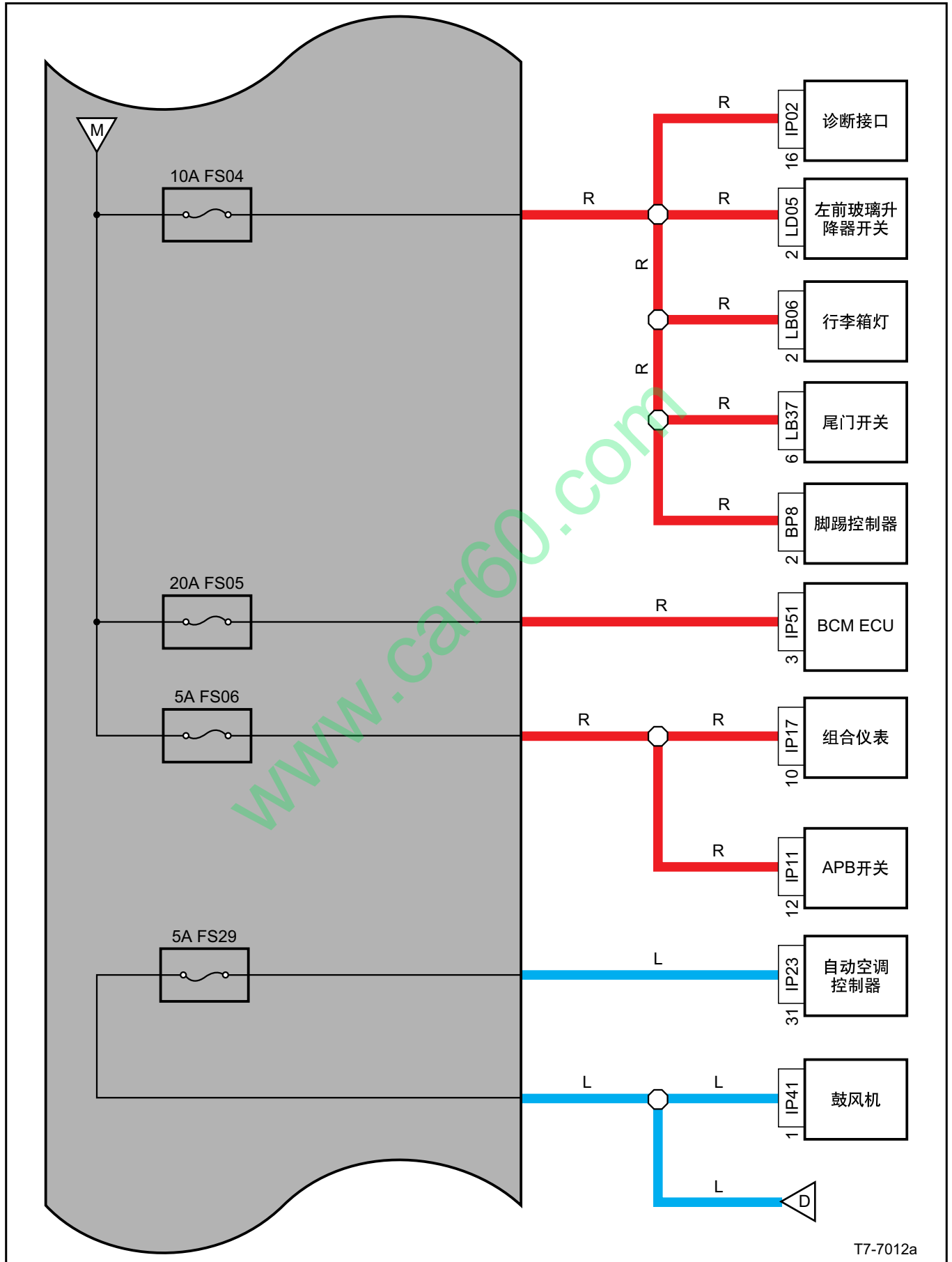
室内保险丝、继电器电源分布图（续2）
