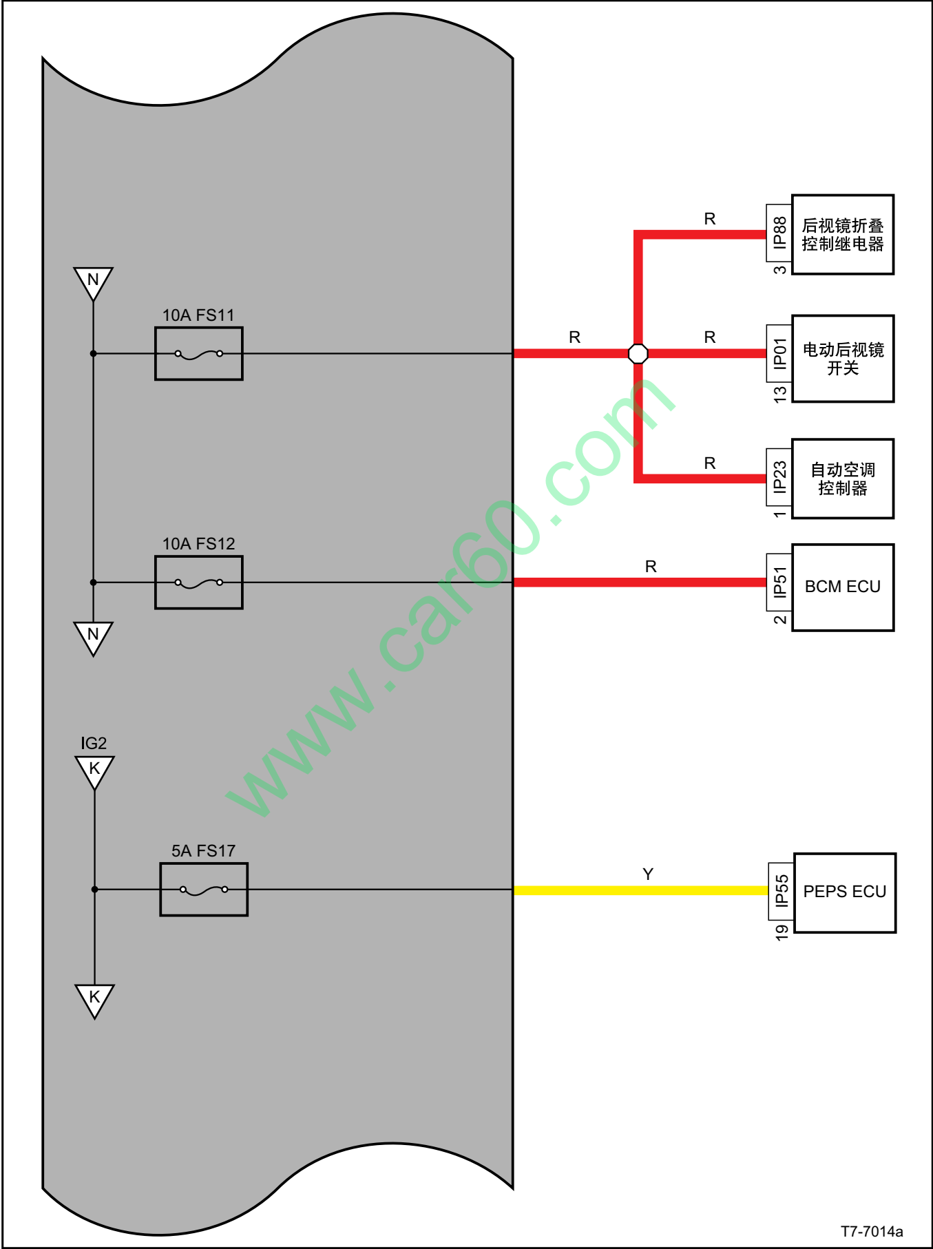
室内保险丝、继电器电源分布图（续4）
