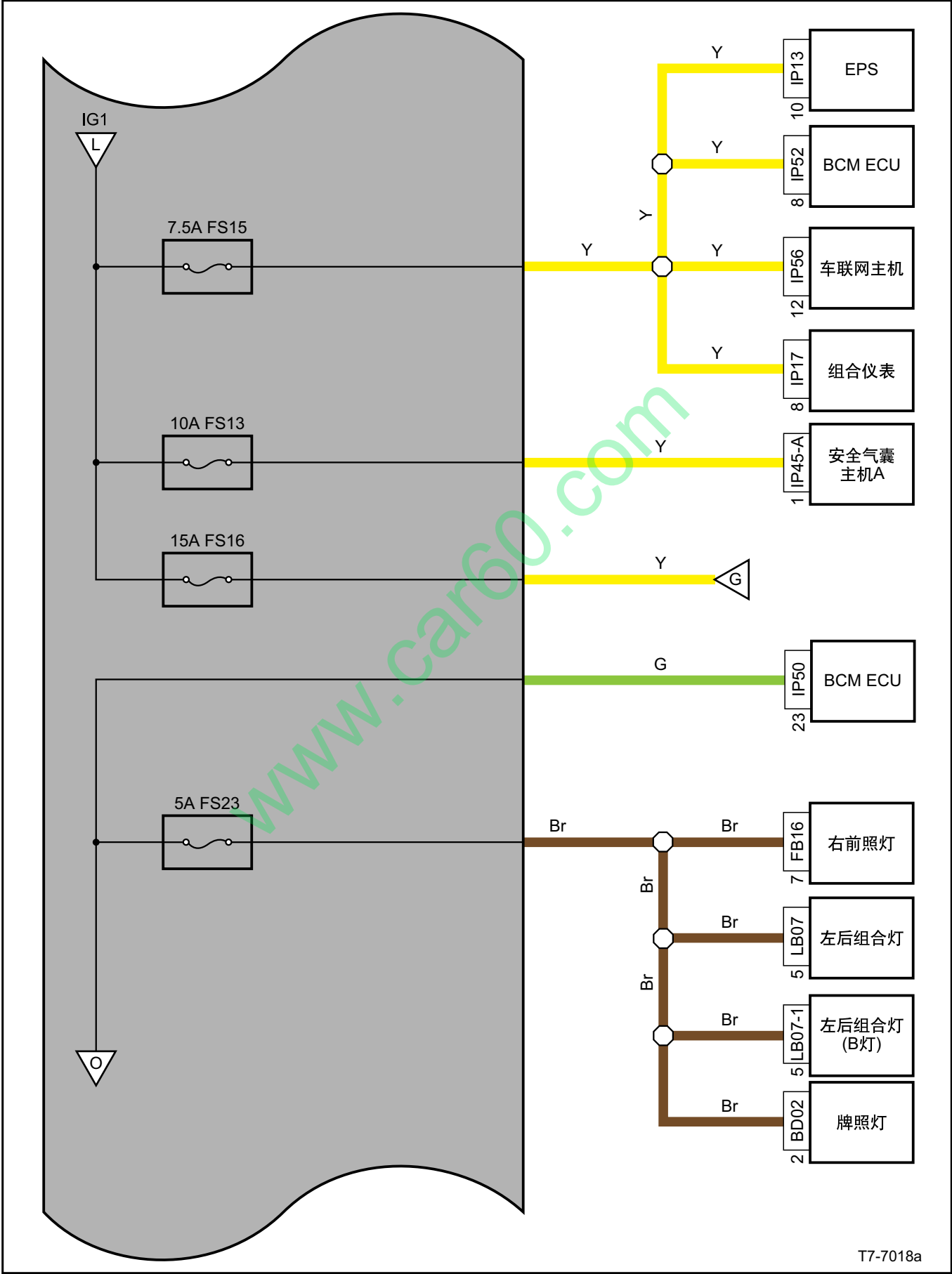
室内保险丝、继电器电源分布图（续8）
