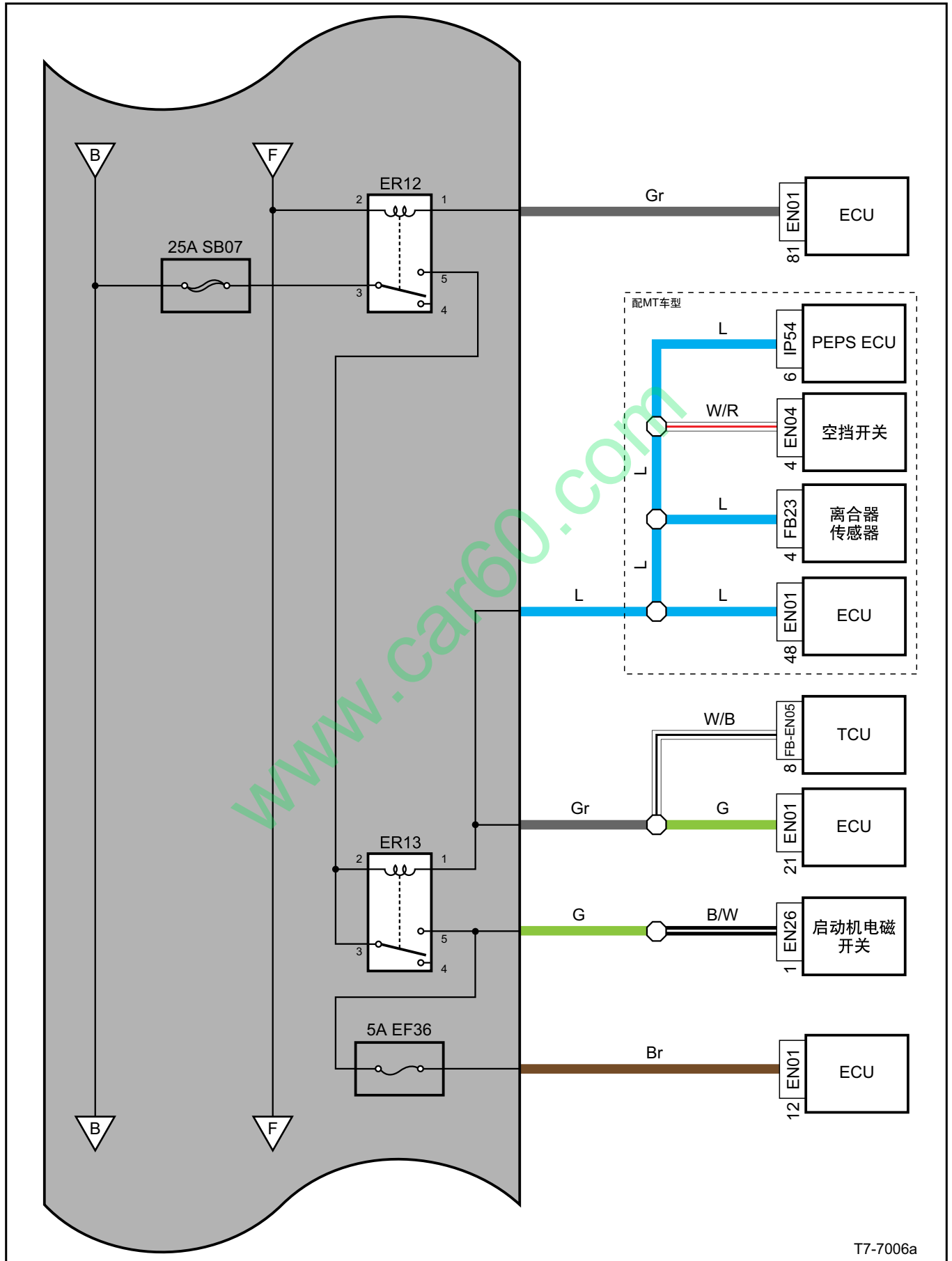
前机舱保险丝、继电器电源分布图 (续5)
