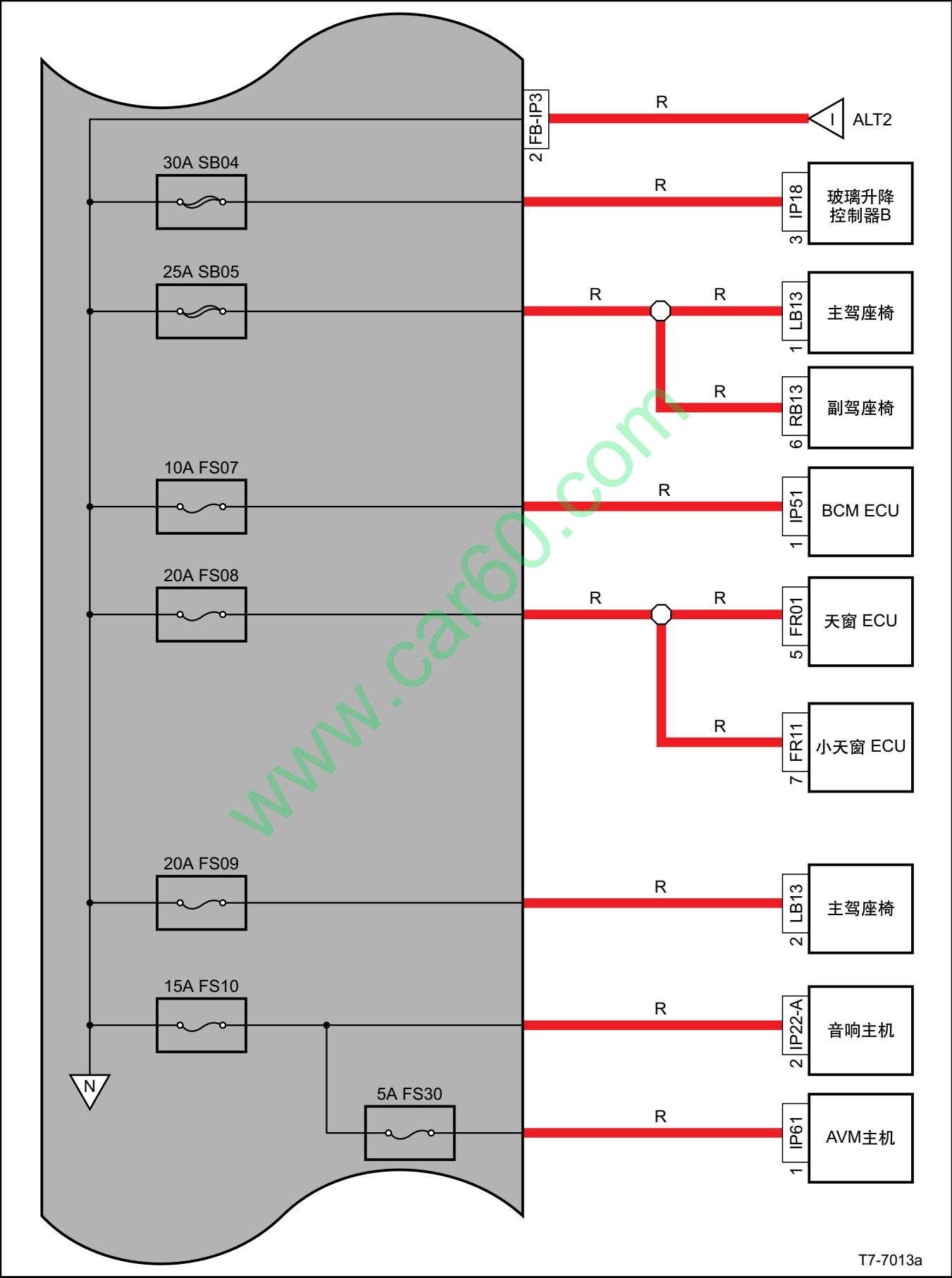
室内保险丝、继电器电源分布图（续3）
