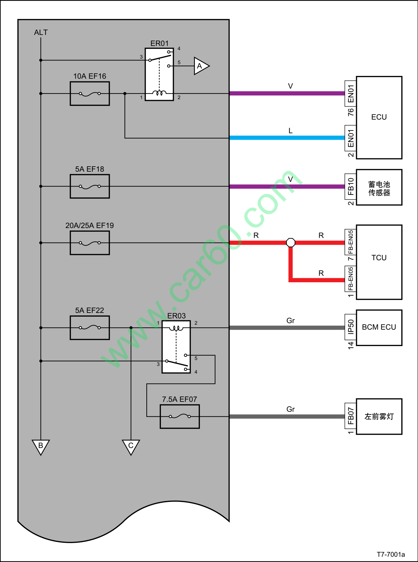
前机舱保险丝、继电器电源分布图
