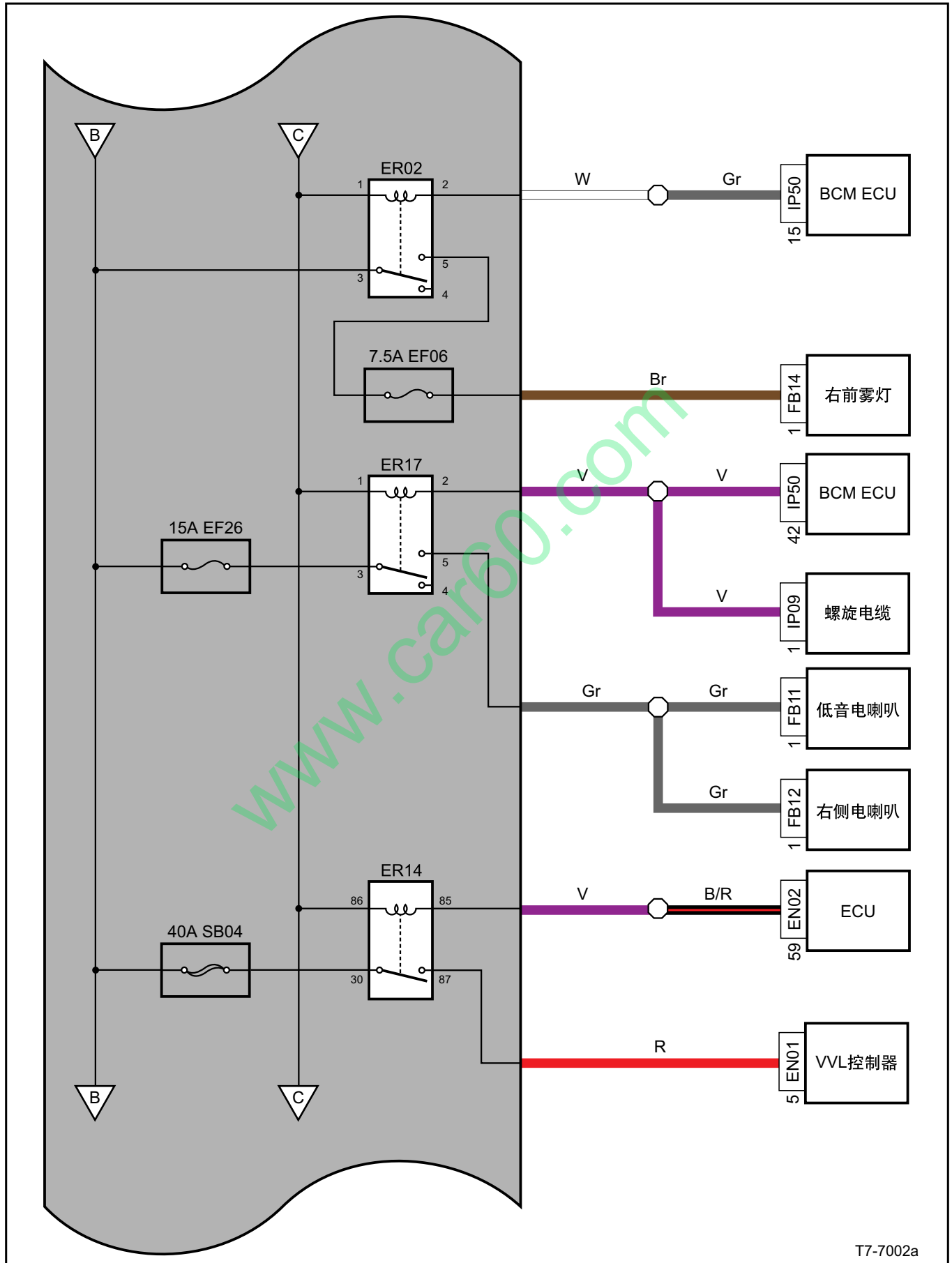
前机舱保险丝、继电器电源分布图 (续1)
