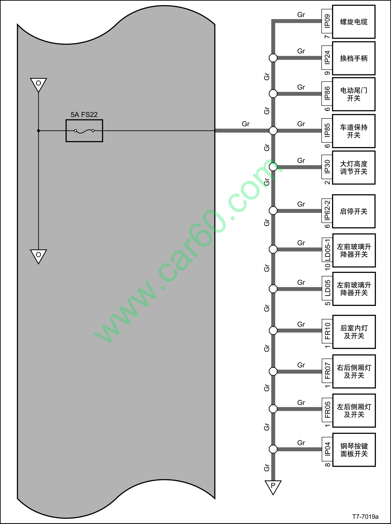
室内保险丝、继电器电源分布图（续9）
