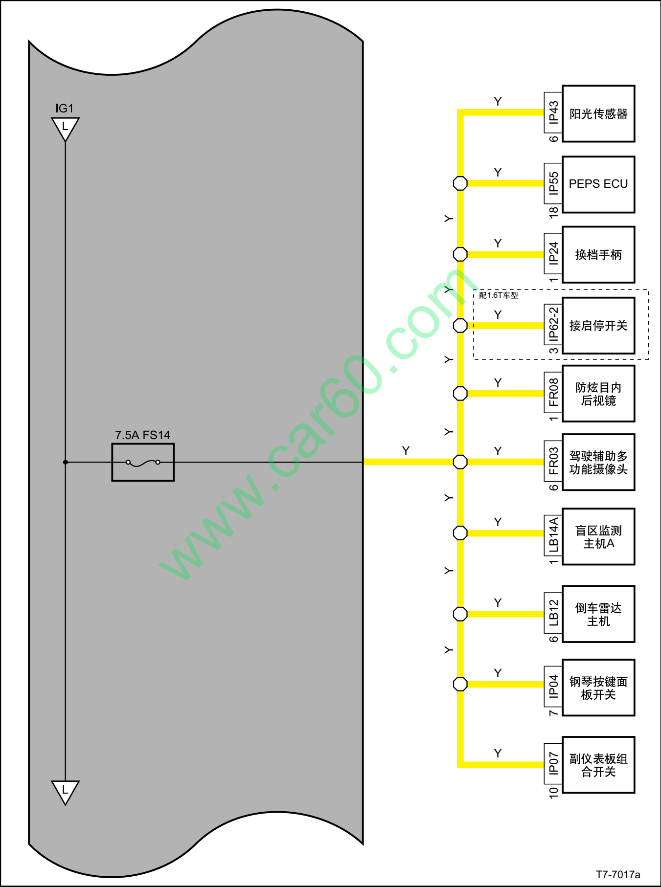
室内保险丝、继电器电源分布图（续7）
