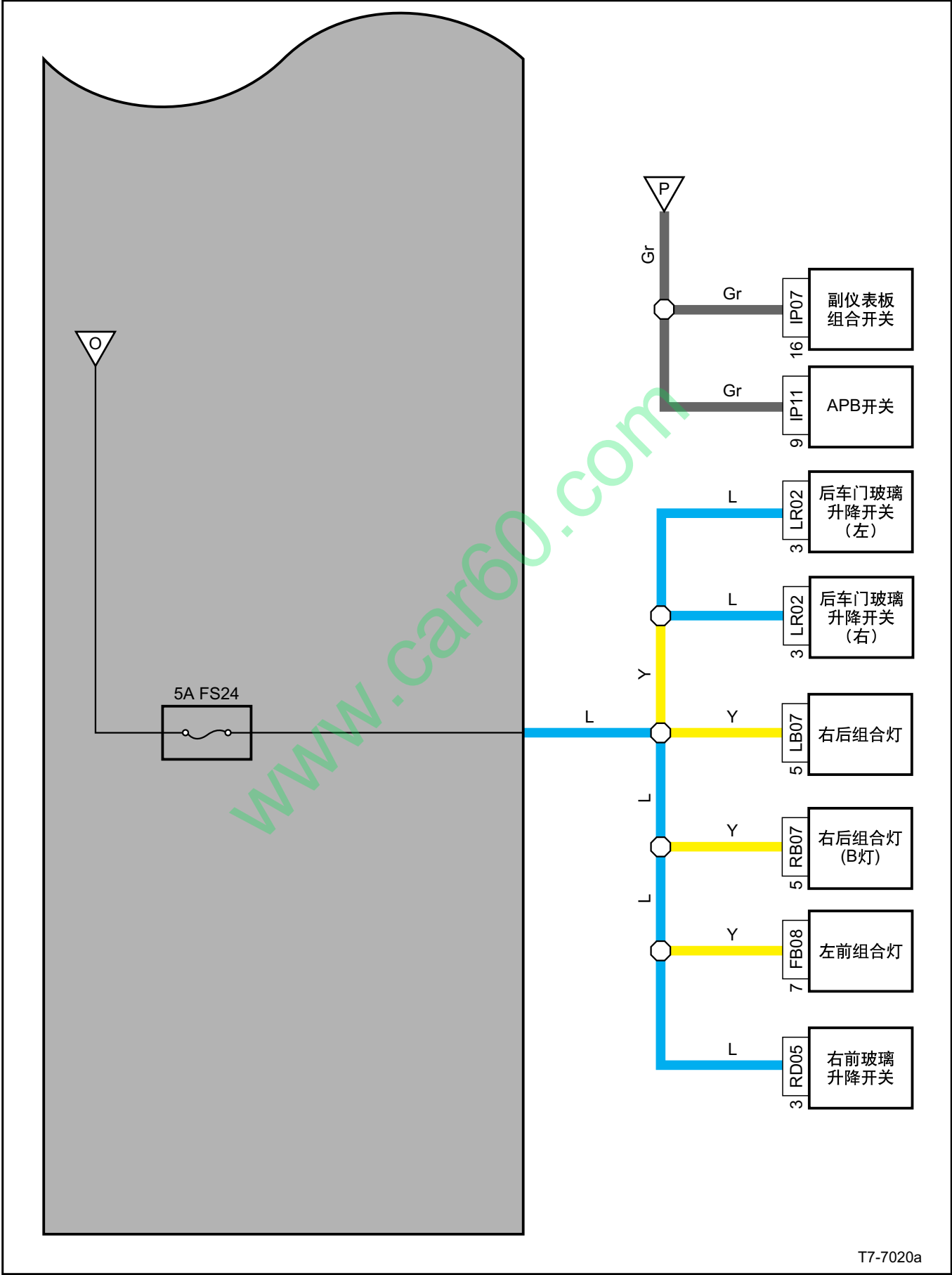
室内保险丝、继电器电源分布图 ( 续10 )
