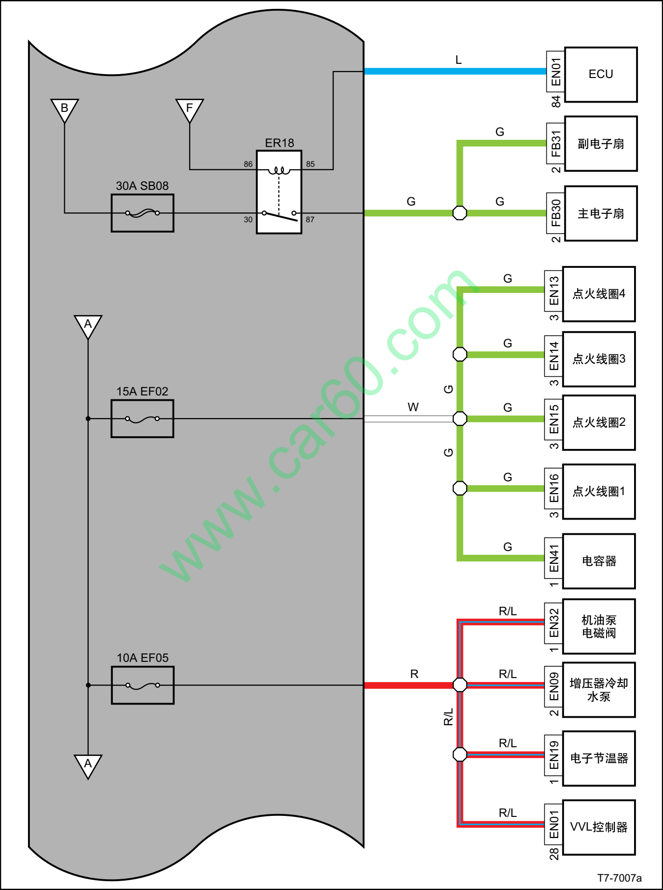
前机舱保险丝、继电器电源分布图（续6）
