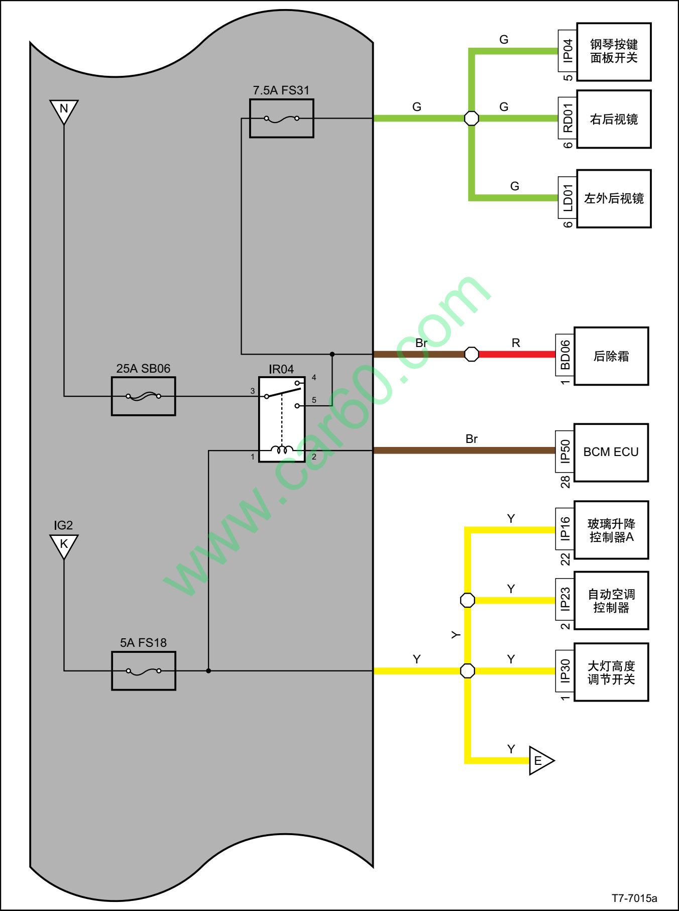
室内保险丝、继电器电源分布图（续5）
