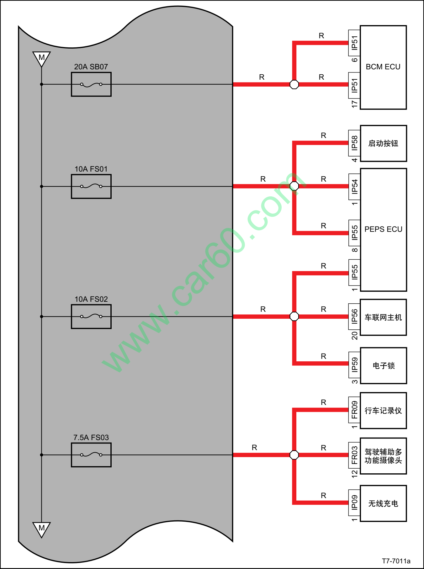
室内保险丝、继电器电源分布图（续1）
