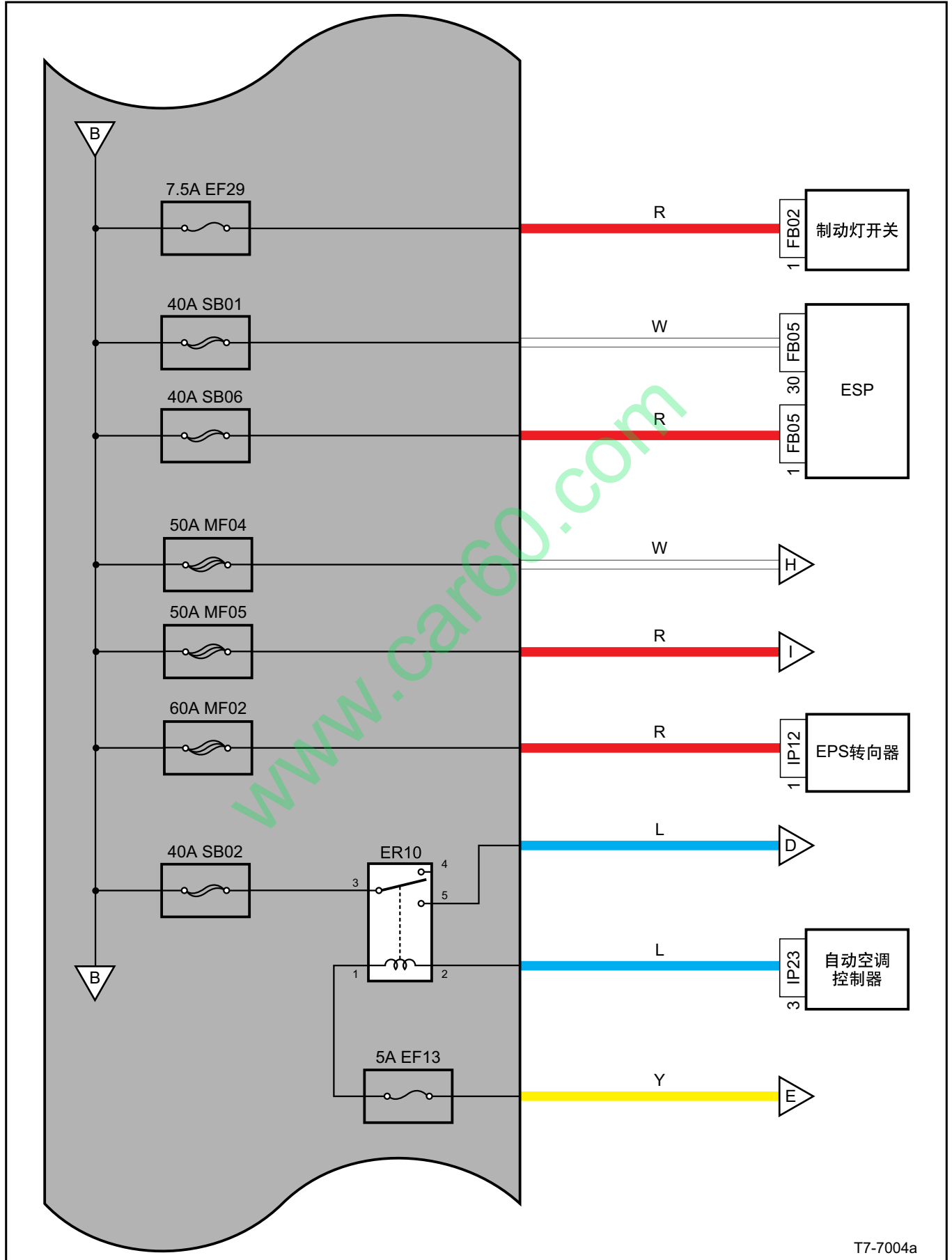
前机舱保险丝、继电器电源分布图（续3）
